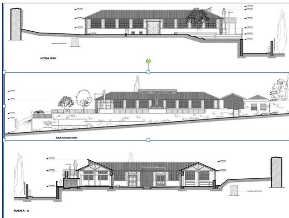
Εργαστήριο της Σχολής Τεχνών και Επαγγελματιών. Σχέδια μελέτης αποκατάστασης
