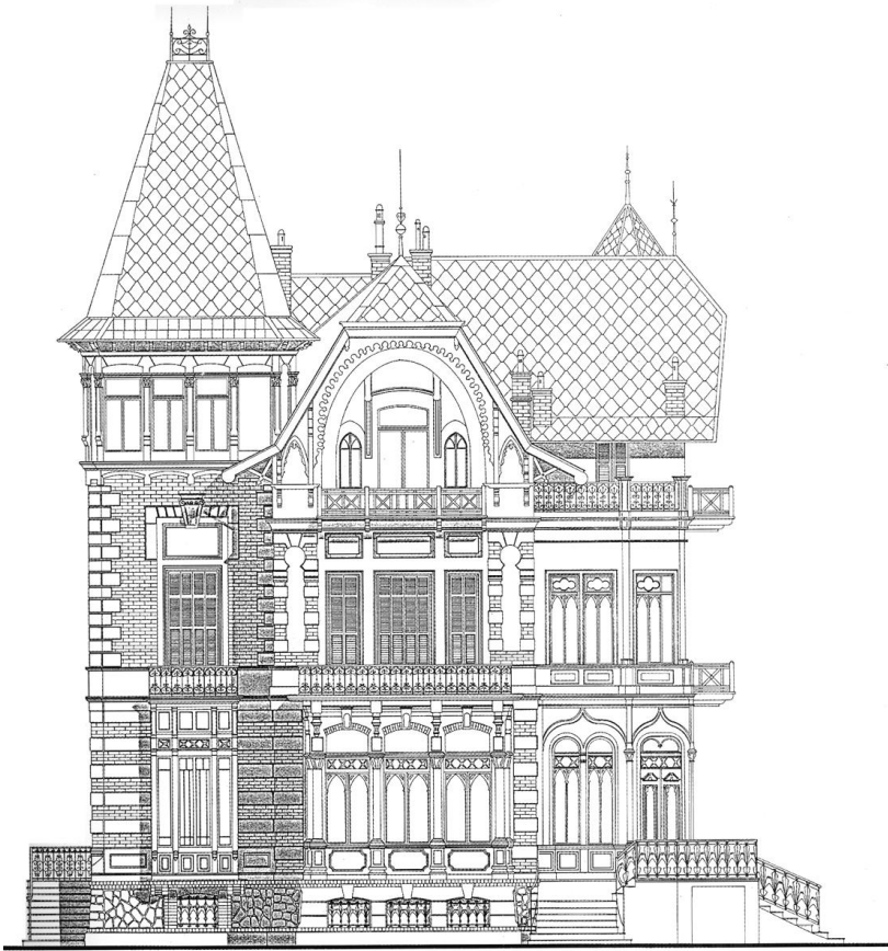
ΣΧΕΔΙΟ ΠΡΟΤΑΣΗΣ ΑΠΟΚΑΤΑΣΤΑΣΗΣ ΔΥΤΙΚΗΣ (ΚΥΡΙΑΣ) ΟΥΧΗΣ.
